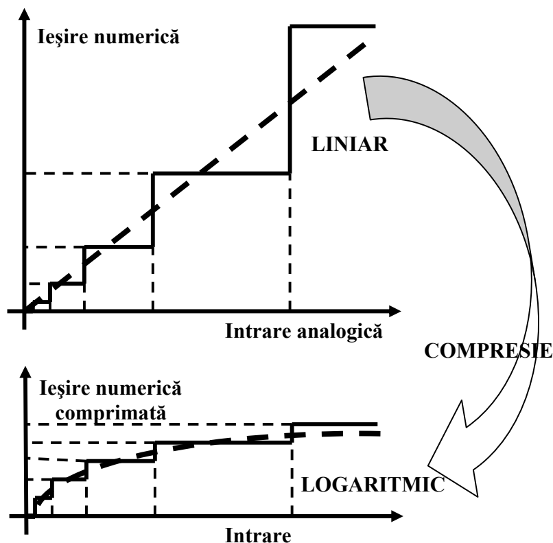
Fig. 3.8. Principiul compresiei.
