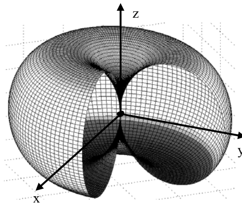
Fig. 2.13. Reprezentarea 3D a caracteristici de directivitate pentru un dipol în \lambda/2 .
