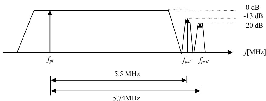
Fig. 6.5. Structura canalului TV în cazul transiterii sunetului pe două canale analogice.
