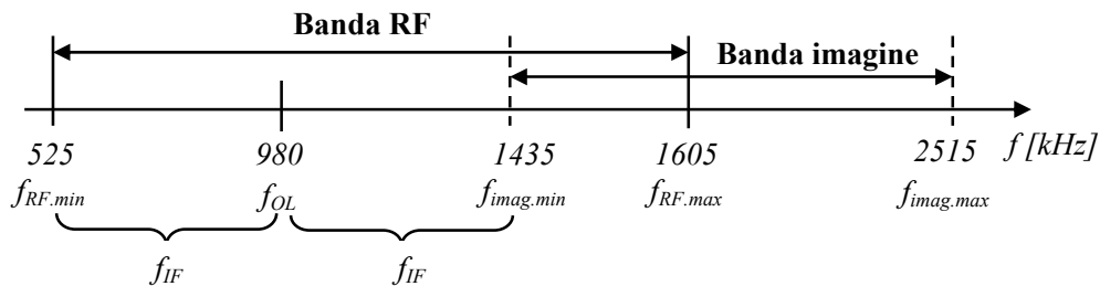
Fig.4.14. Banda frecvențelor imagine pentru gama radio AM.
