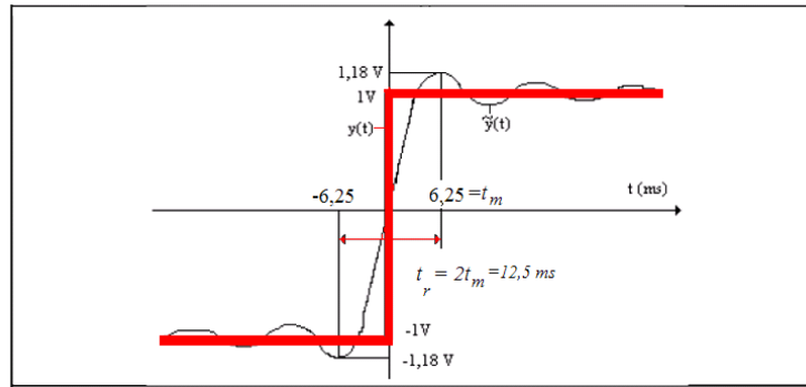
Fenomenul Gibbs pentru o undă rectangulară cu T_0=1\text{ s} (factor de umplere 0,5).
