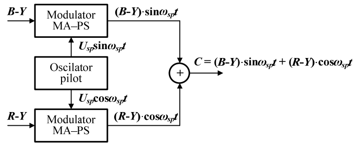
Fig. 7.1. Principiul modulației de amplitudine în cuadratură.
