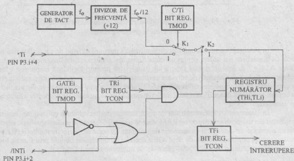
Fig.8.14. Structura unui circuit numărator/temporizator ( N/T_i ; i = 0 sau 1 ).
