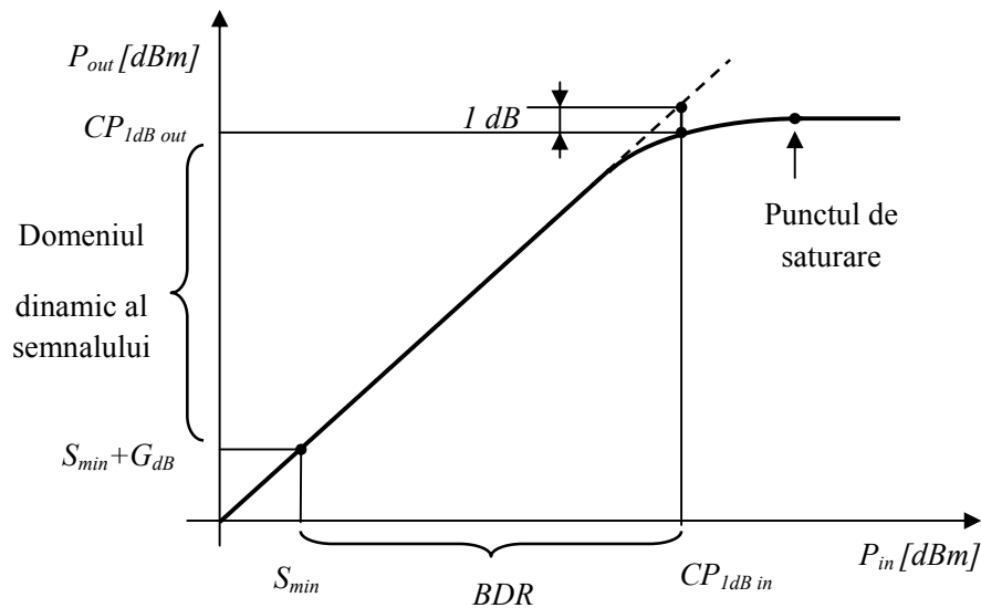
Fig.4.43. Definirea BDR .
